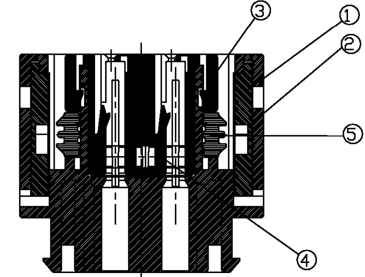
SECT A-A
